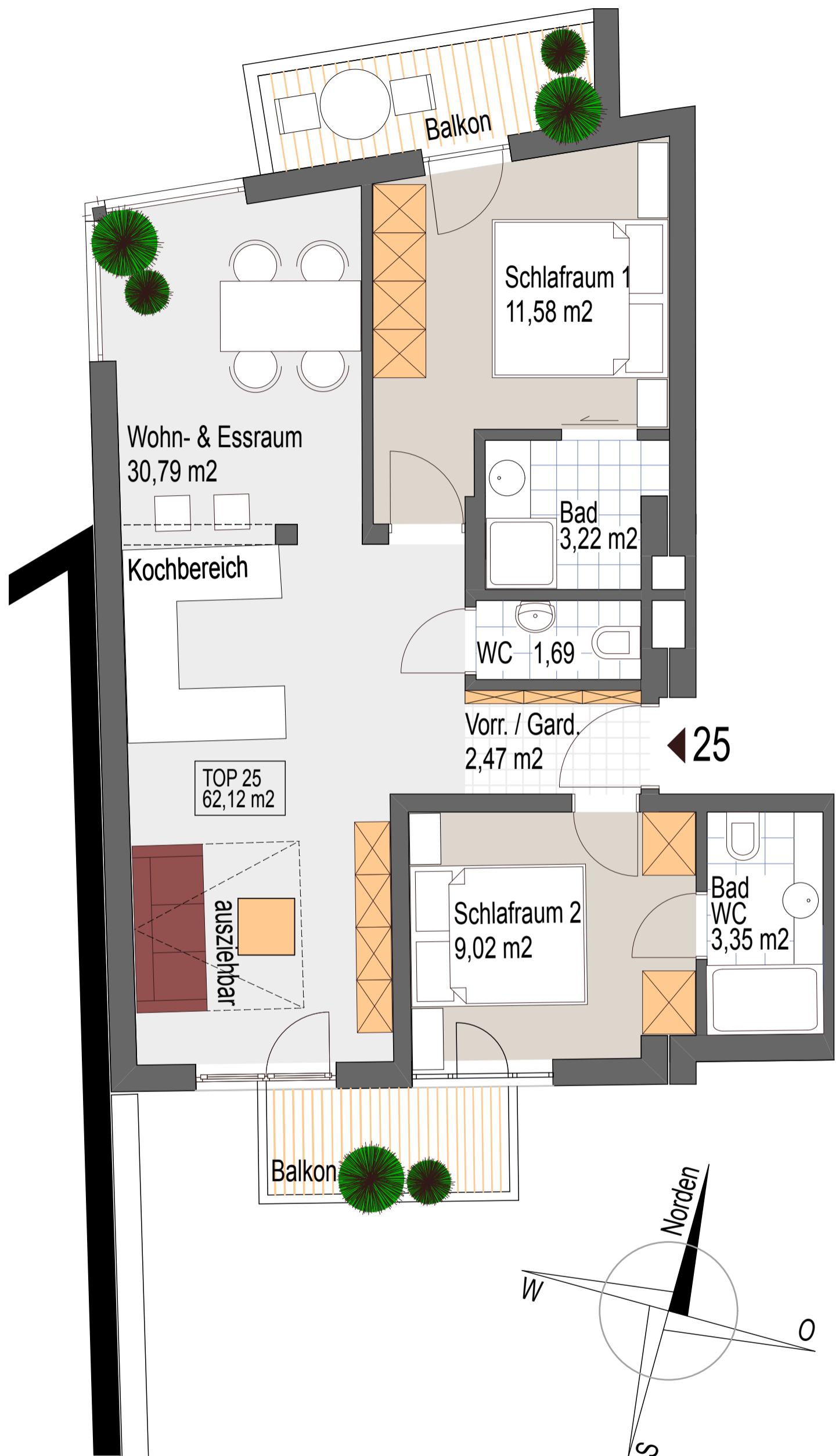
Wohnung 25 im 2. OG M 1:50
