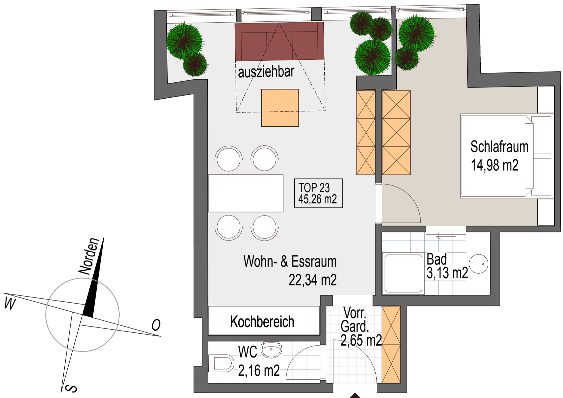
Wohnung 23 im 2. OG M 1:50
