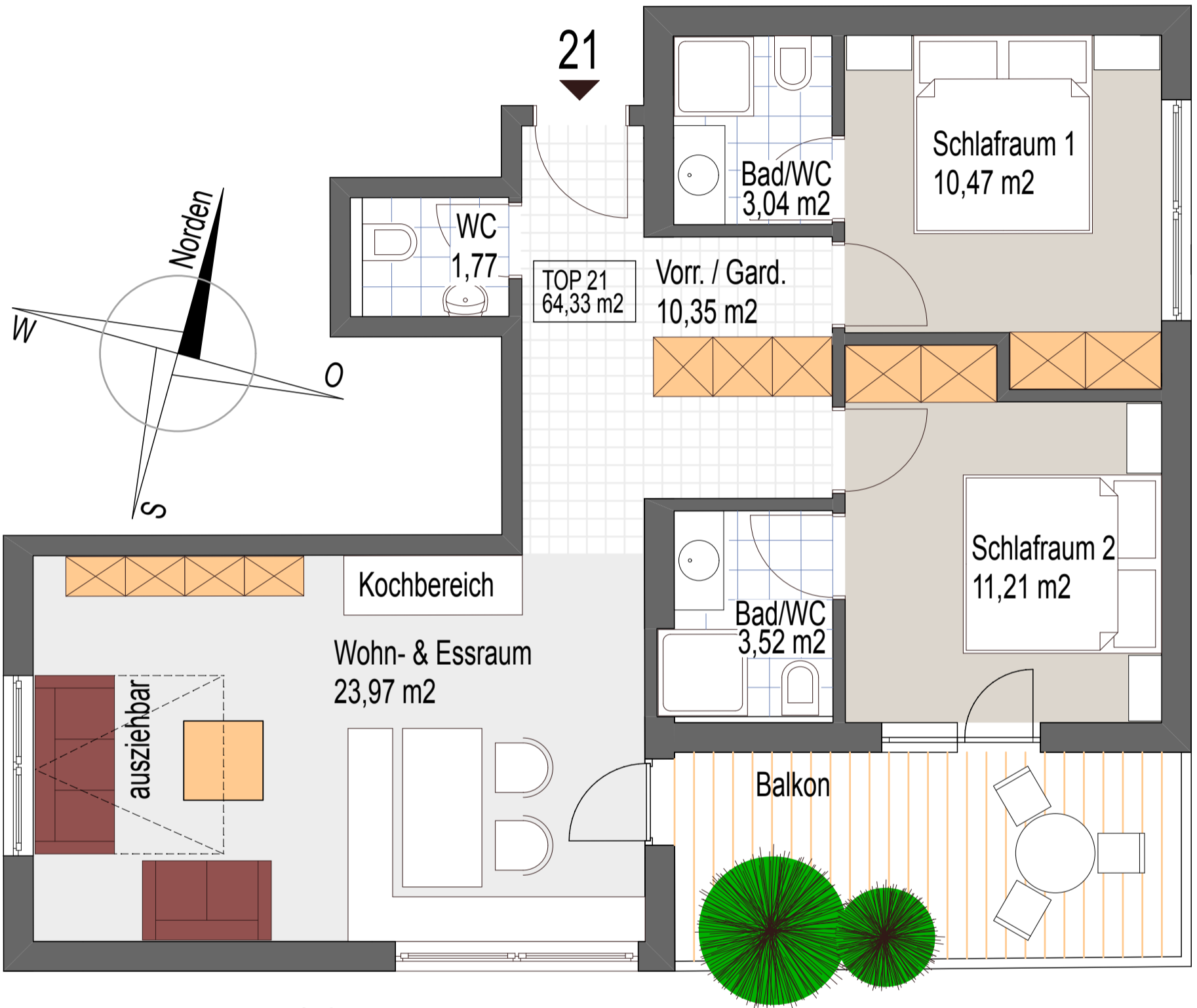
Wohnung 21 im 2. OG M 1:50
